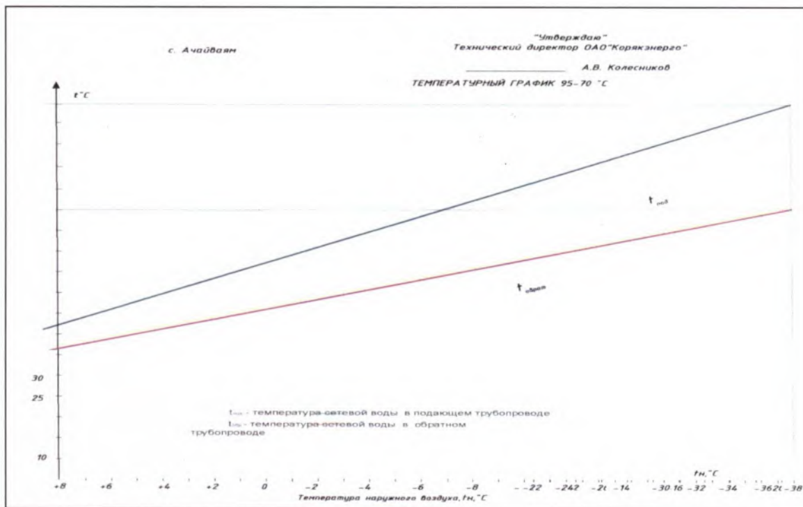
Рис.2.1.3. Температурный график отпуса теплоносителя
